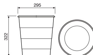
CESTINO GETTACARTE WASTEPAPER BASKET
